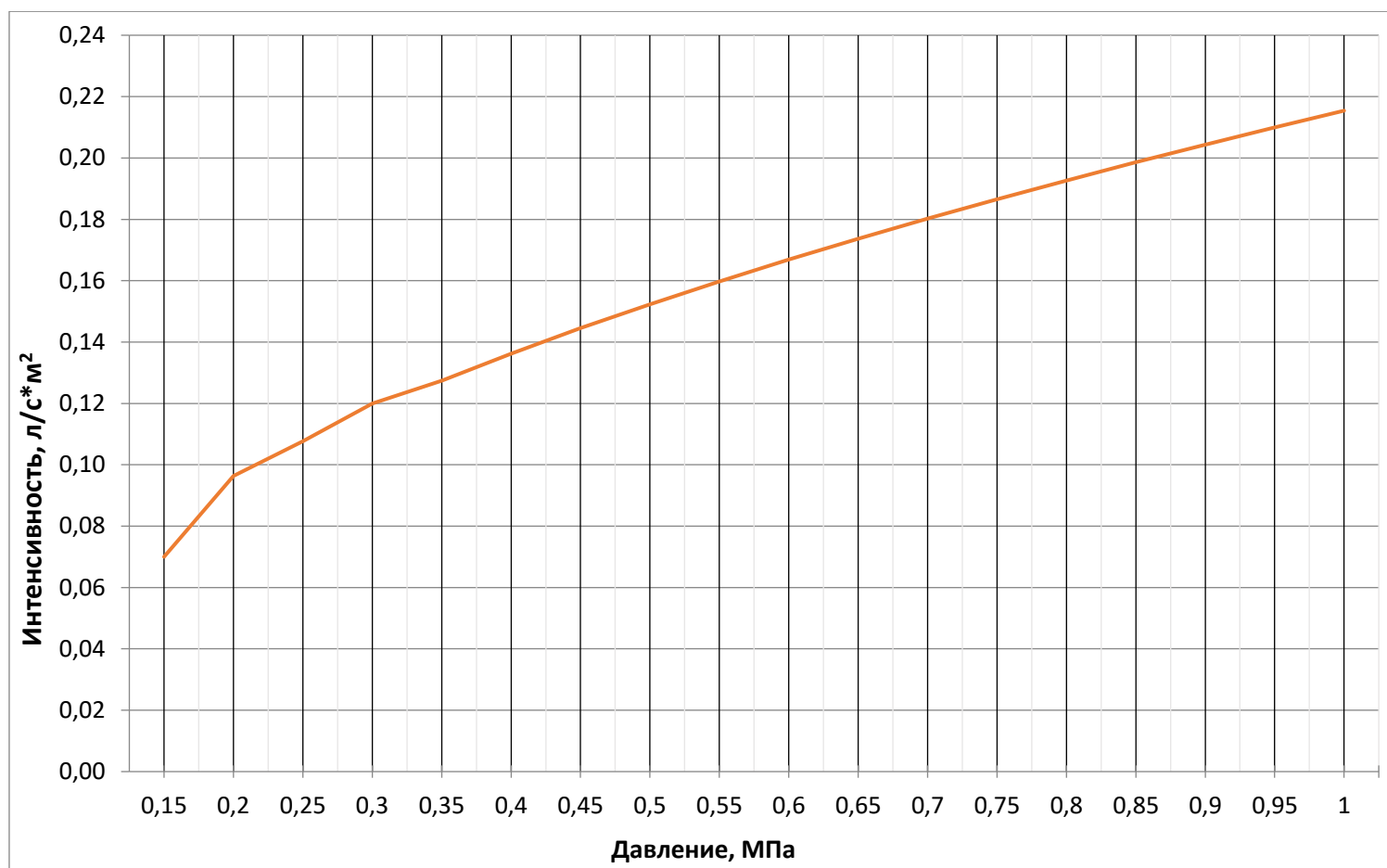
График зависимости интенсивности орошения пеной для высоты 2,5 м и площади 3х4 м 2
