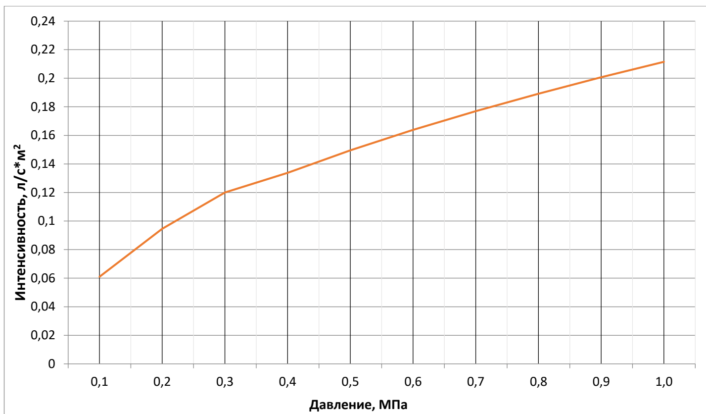
График зависимости интенсивности орошения водой для высоты 2,5 м и площади 3х4 м 2
